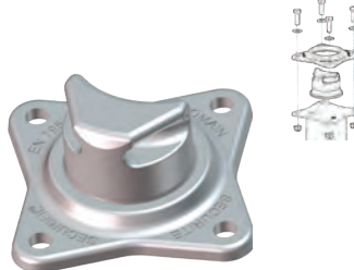
Renvoi d'angle alu orientable Tous les 15 mètres maximum 4 trous entraxe 100 mm
