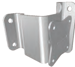
Equerre réglable en acier galvanisé pour renvoi d'angle orientable Permet d'installer un renvoi d'angle dans un angle mural intérieur ou extérieur 2 fixations M12
