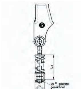
Type D : boite à coin + piton équipé avec ressort
