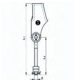
Type AM : boite à coin + piton équipé
