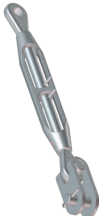
Tendeur inox oeil/chape Pour régler la tension de la ligne de vie lors de l'installation
