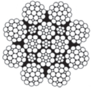
Câble double parallèle
