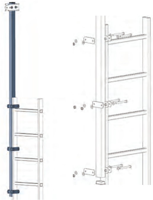
Mat d'extension à brider sur échelle Fixé sur un montant de l'échelle
