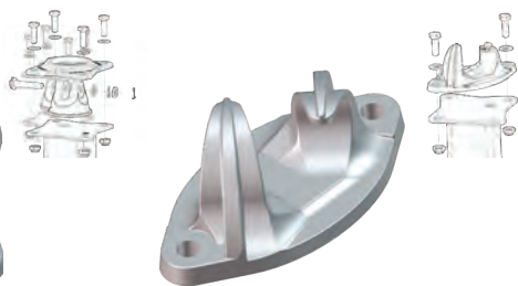
Intermédiaire alu Tous les 15 mètres maximum 2 trous entraxe 100 mm Fixations M10 ou m12
