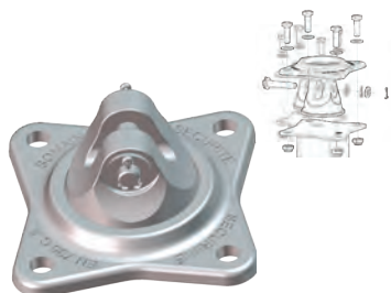
Extrémité alu orientable 4 trous entraxe 100 mm Fixations M10 ou m12
