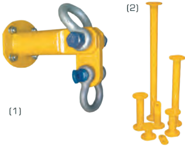
(1) Paire des sous-ensembles d'extrémités équipée de manilles lyres - Réf. MSED (2) Entretoise avec visserie - Réf. ME
