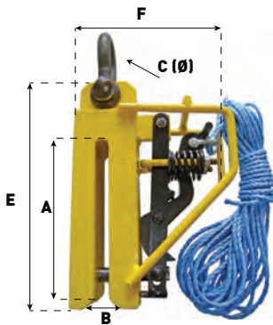
Pince palplanche
