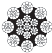
Câble avec infiltration plastique
